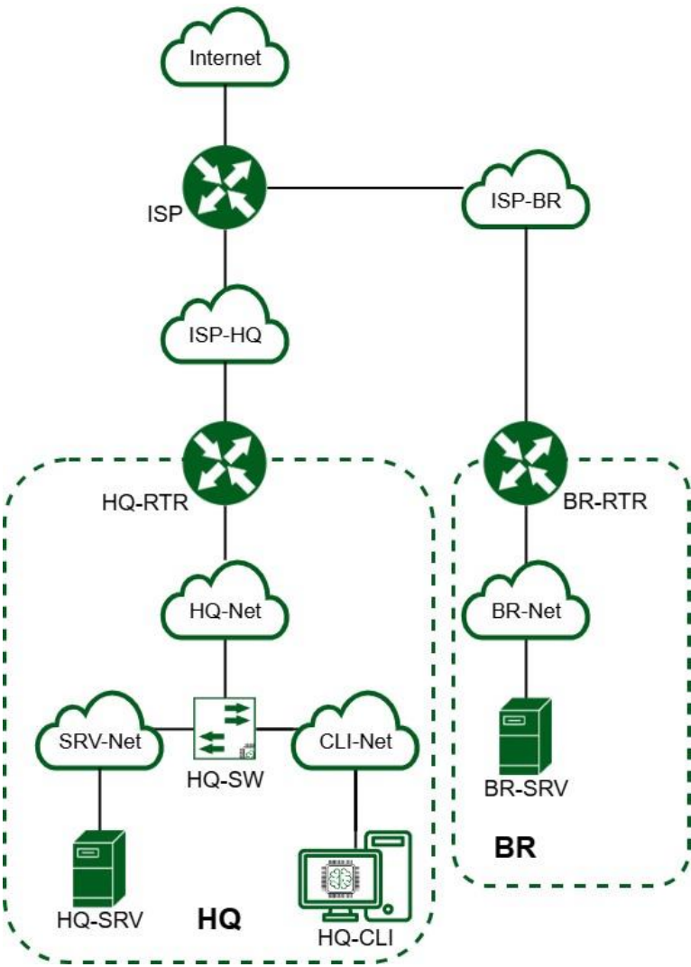
Рисунок 2. Топология сети
