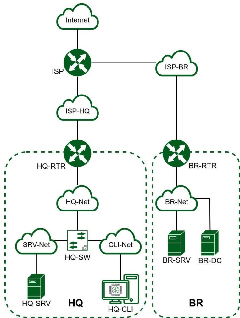
Рисунок 3. Топология сети
